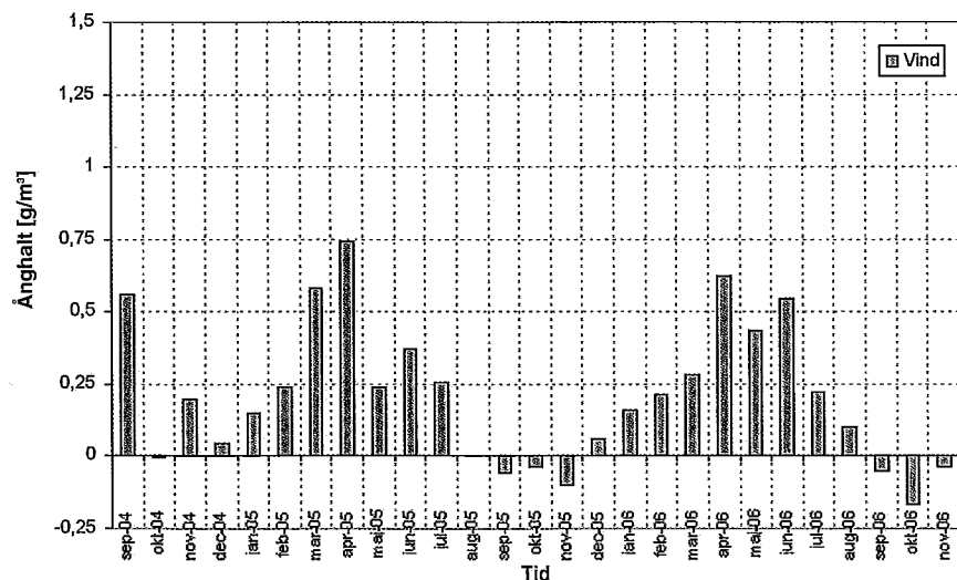
Figur 7: Månadsmedelvärde för fuktillskott (g/m 3 ) på vinden.
